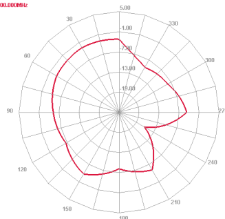
E2 Face 2400.000MHz
