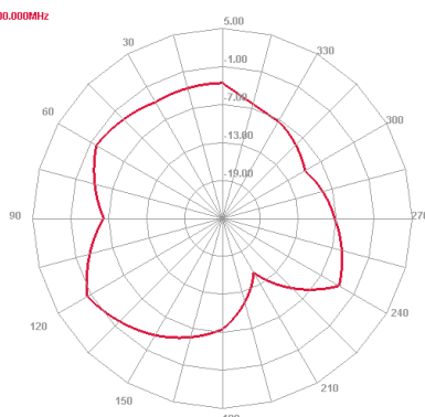
E2 Face 4800.000MHz
