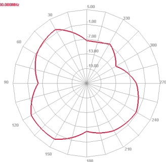
Horizontal 2400.000MHz
