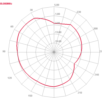
Horizontal 3500.000MHz
