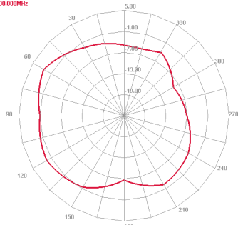
E2 Face 3500.000MHz
