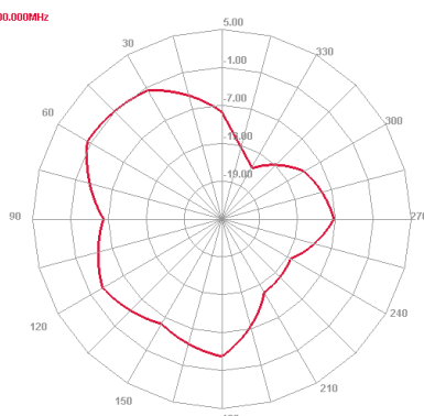
Horizontal 4800.000MHz
