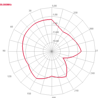
E2 Face 2400.000MHz
