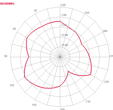
E2 Face 4800.000MHz
