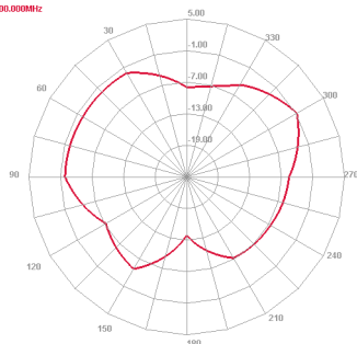
E2 Face 2600.000MHz
