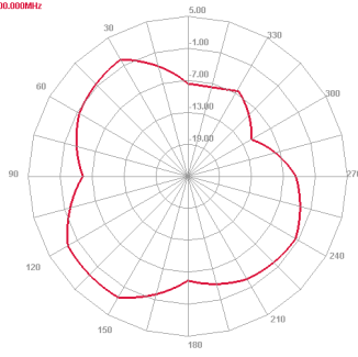
Horizontal 2400.000MHz
