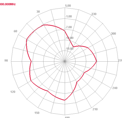
Horizontal 4800.000MHz
