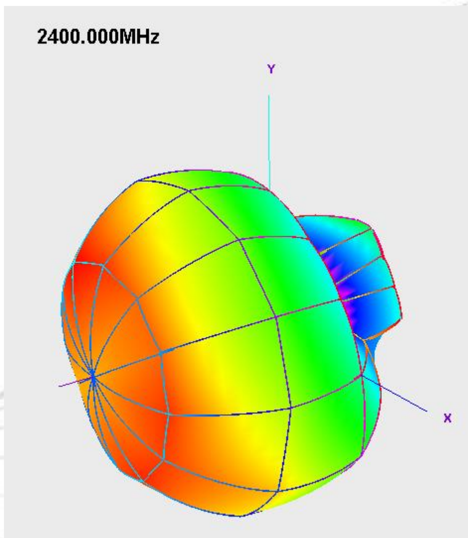
实测方向图 2.4GHz
