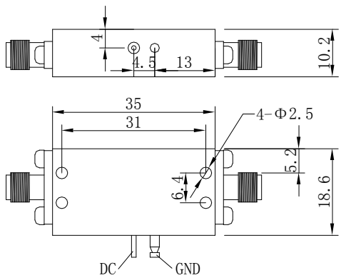
UNIT:mm XB-02A
