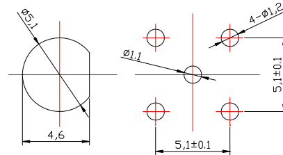
安装开孔尺寸图
