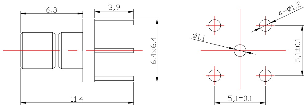
安装开孔尺寸图
