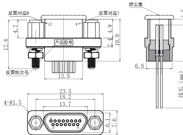
(去掉防尘盖 插合面视图)
